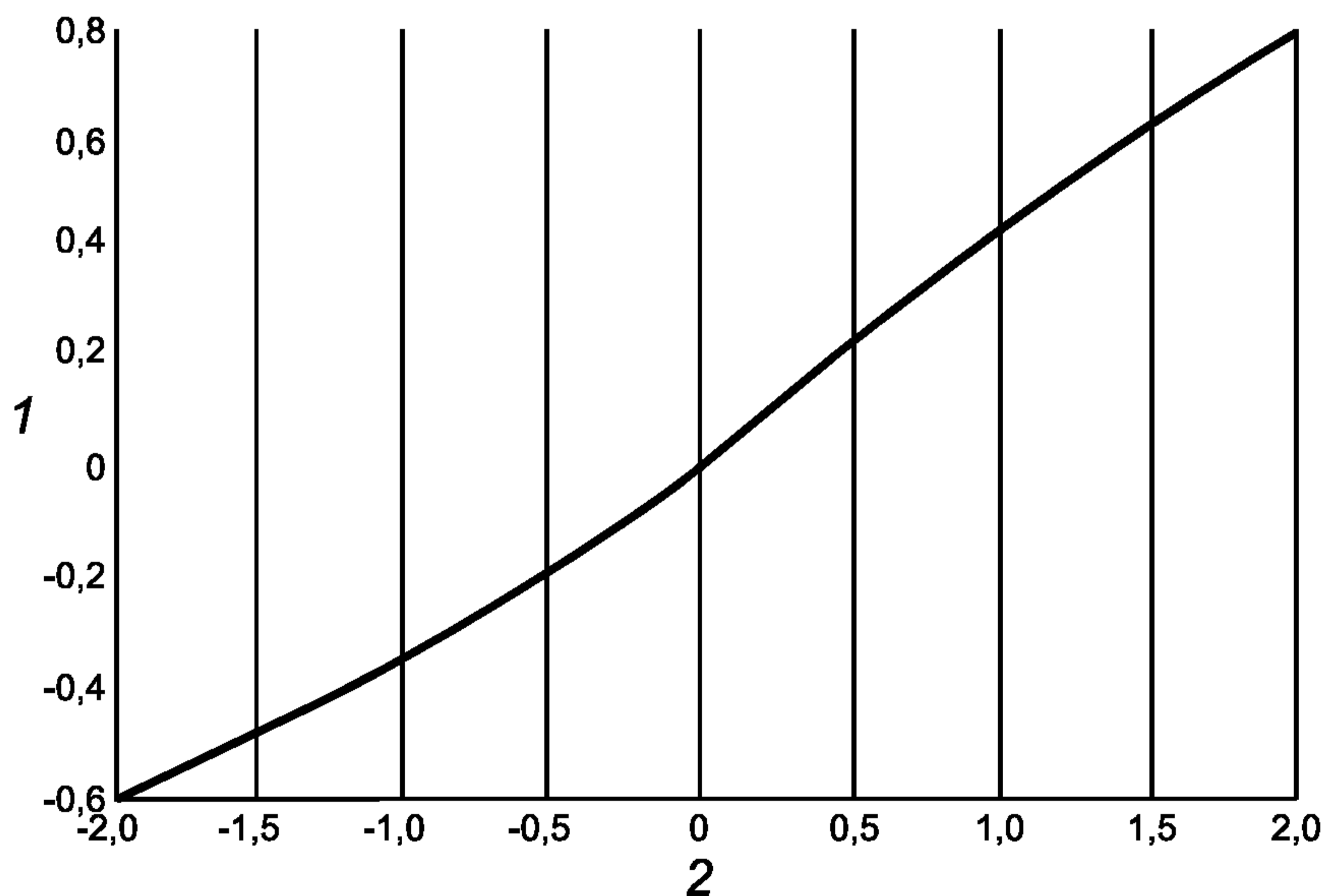
1 — влияние на холодную воду, К; 2 — атмосферный градиент, К на 100 м
