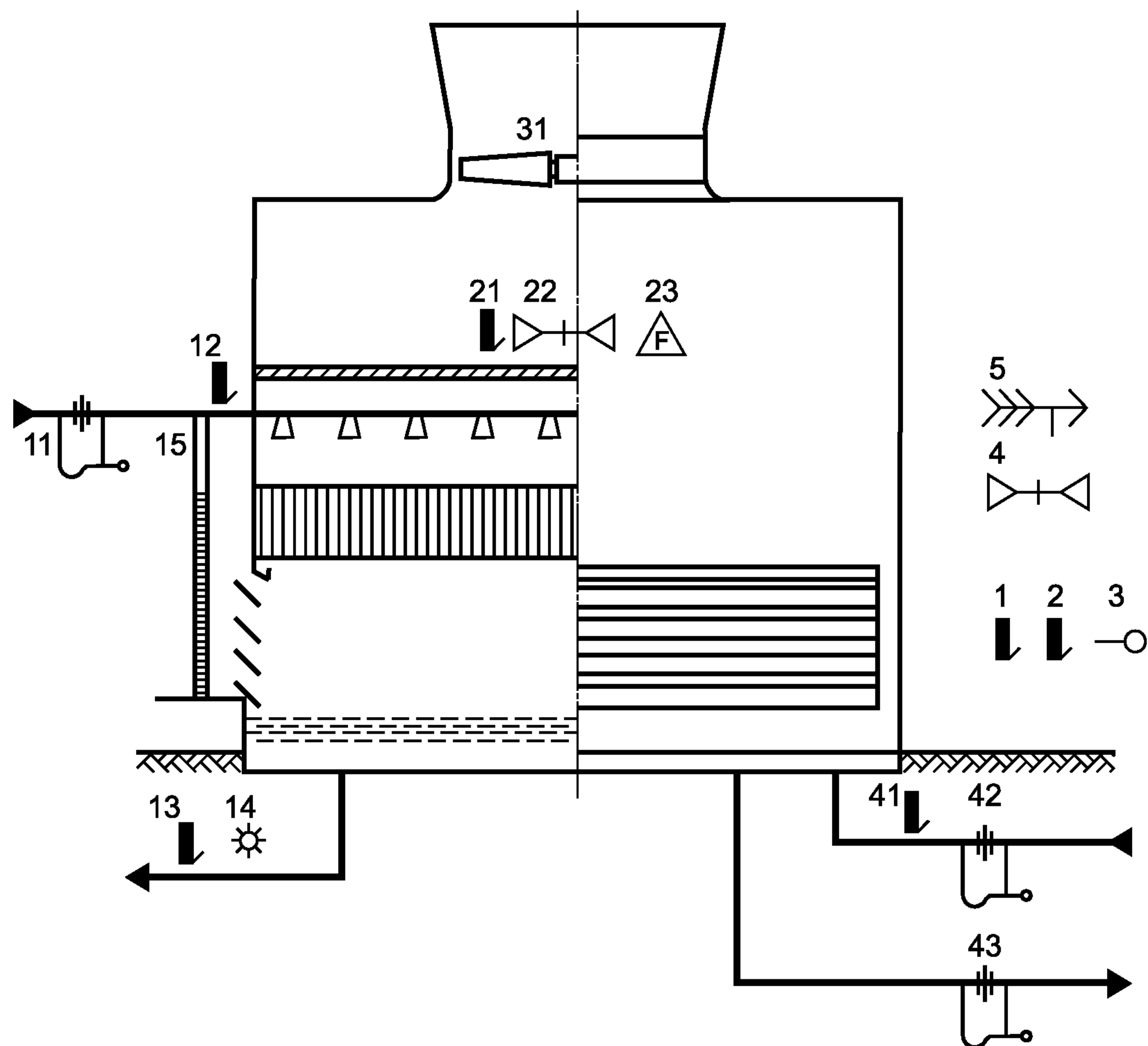
Рисунок 4 — Расположение точек измерений в вентиляторной градирне
