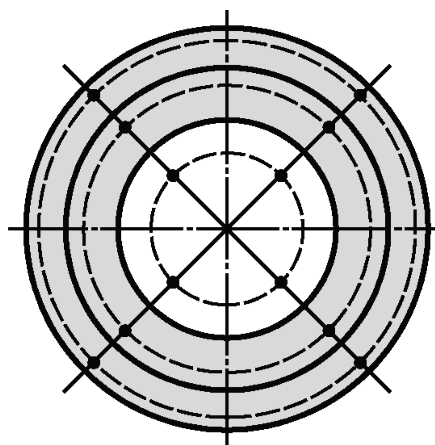
Рисунок 2 — Пример секционирования измеряемой зоны (круговая зона)
