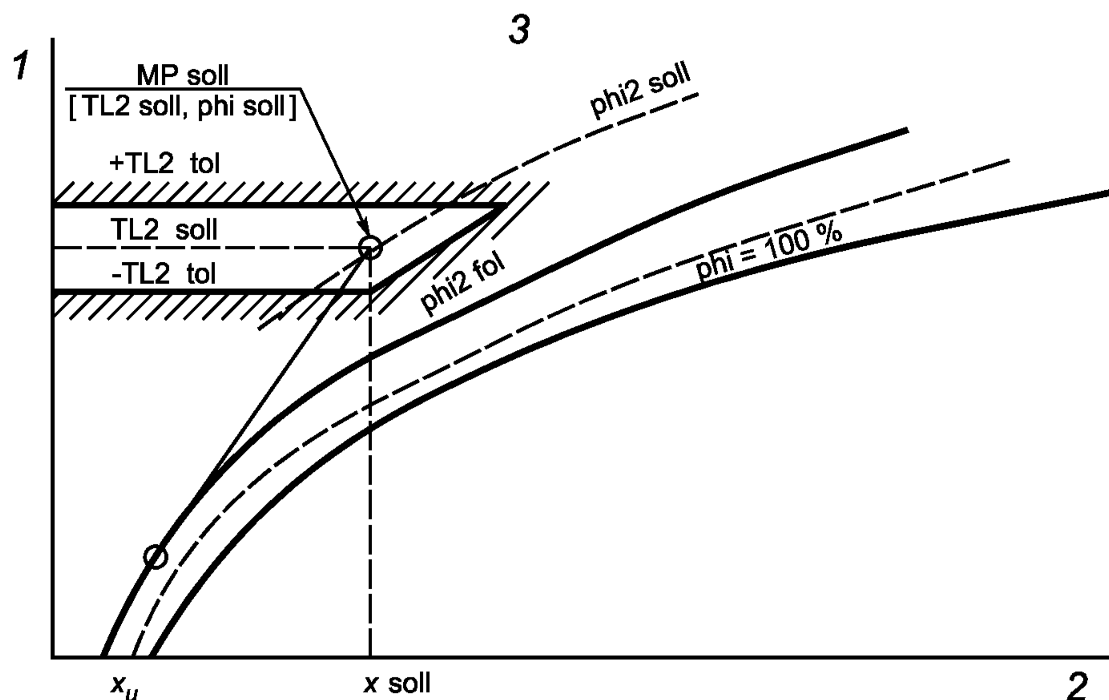
1 — массовая энтальпия воздуха h ; 2 — абсолютная влажность окружающего воздуха x\varphi ; 3 — диаграмма Молльера
