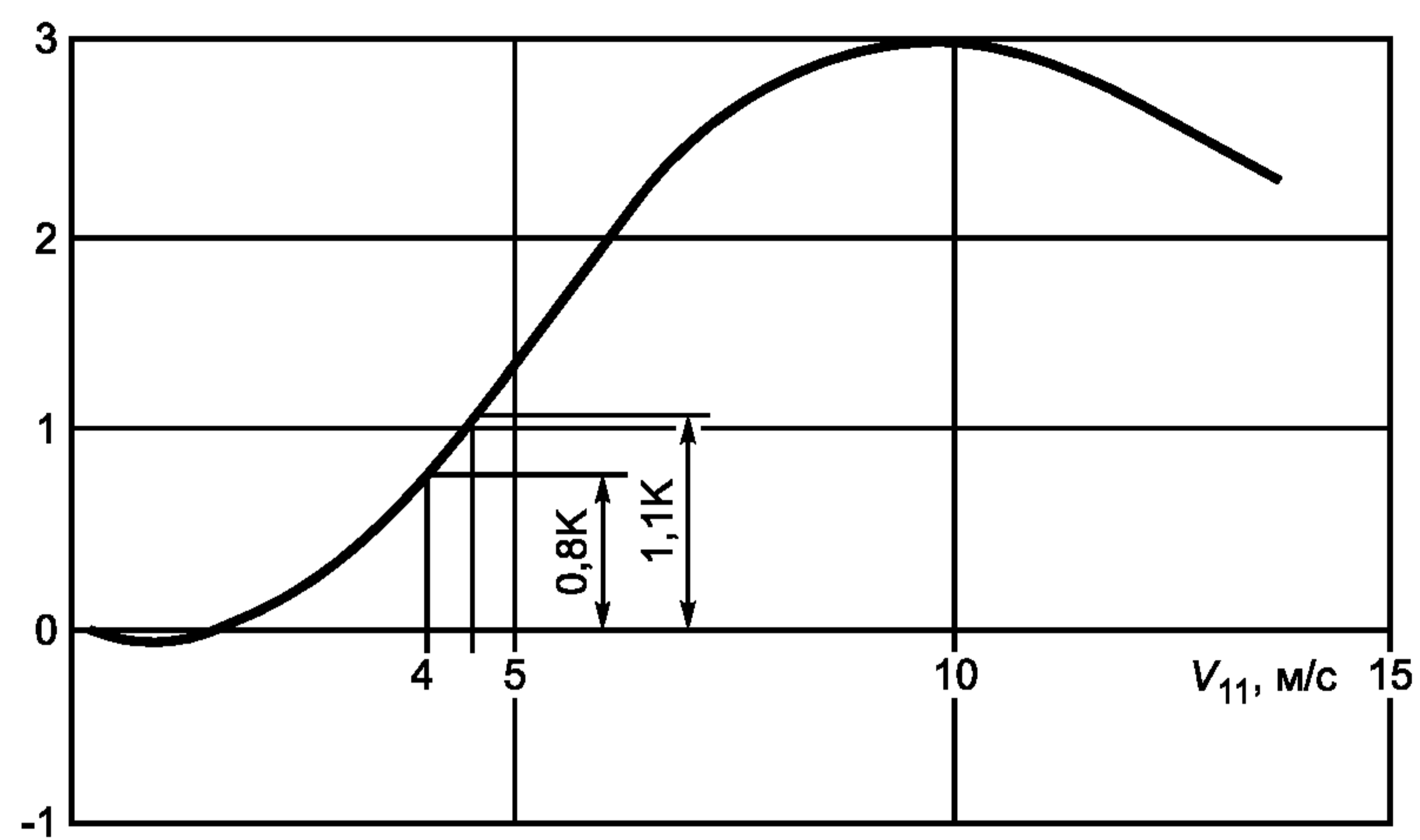
Рисунок А.2 — Пример воздействия ветра на градирню с противотоком и естественной тягой
